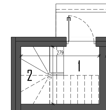
RZUT PARTERU
