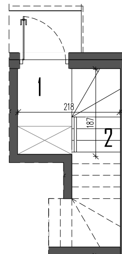
RZUT PARTERU
