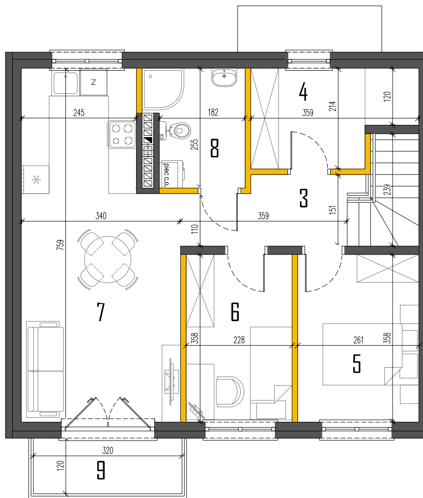
RZUT PIĘTRA
