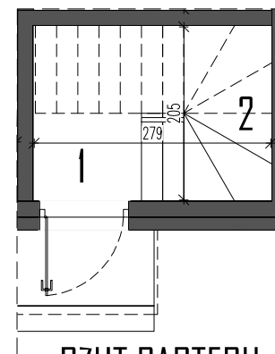
RZUT PARTERU
