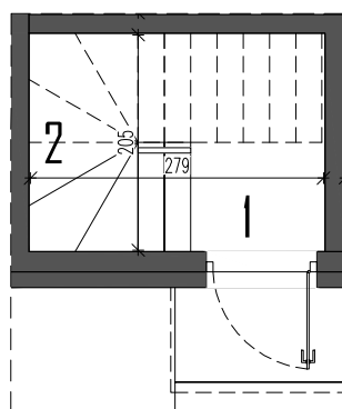
RZUT PARTERU
